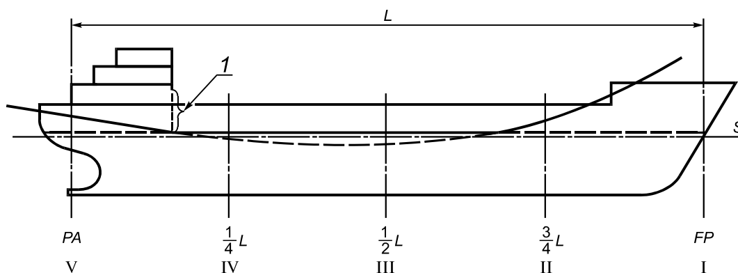
1 — дополнительная ордината для круглых иллюминаторов, расположенных в лобовых переборках
