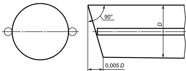
Рисунок 6 — Предельный перекосяк плоскости торца шпунтового профиля
