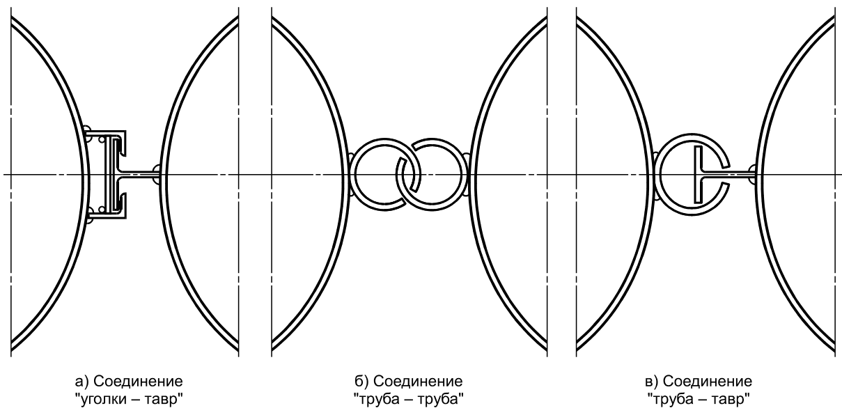
Рисунок 3 — Предпочтительные типы замковых соединений шпунтовых профилей
